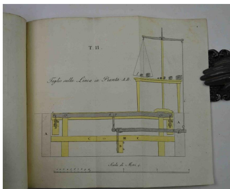
ROSA LUIGI. Della nuova bilancia a ponte a cinque leve. Milano, 1821 (vedi scheda completa nel catalogo)
